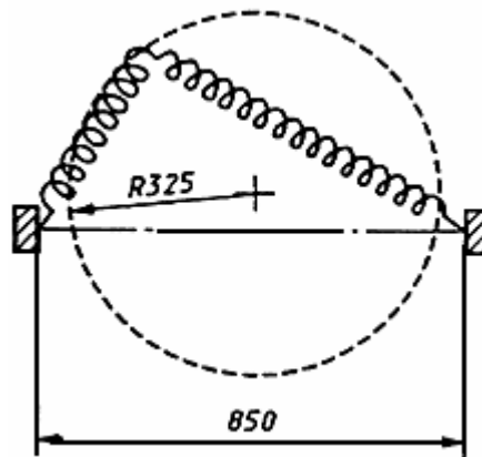
Рисунок 2 - Схема установки для испытания износостойчивости спиральных шнуров
