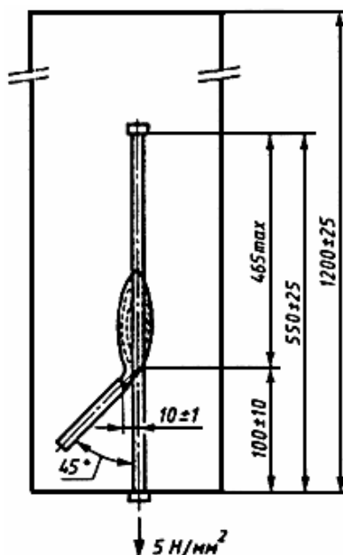
Рисунок Е.1 - Испытательная камера
